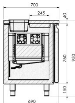
SEZIONE C-C
