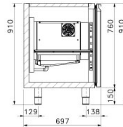
SEZIONE B-B
