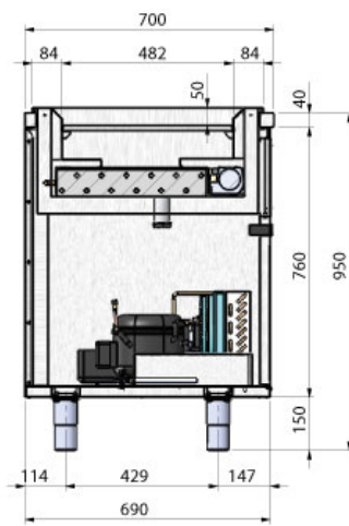
SEZIONE E-E
