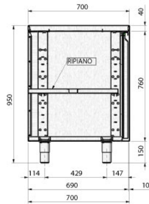
SEZIONE D-D
