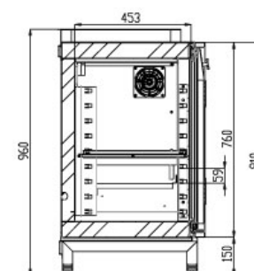
SEZIONE B-B
