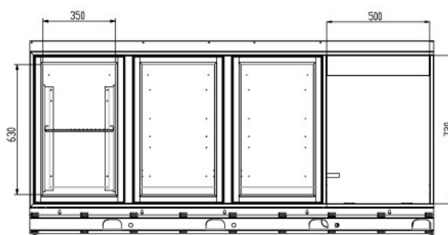
SEZIONE B-B
