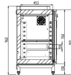
SEZIONE B-B
