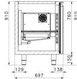
SEZIONE B-B
