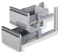
66157311 (1/2-1/2) 66157344 (1/3-2/3) Bloc tiroirs détaché H660
