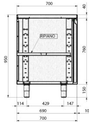
SEZIONE D-D
