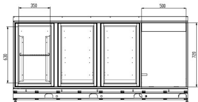
SEZIONE B-B
