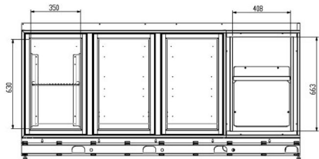
SEZIONE B-B
