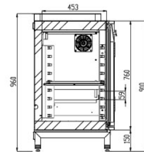
SEZIONE B-B
