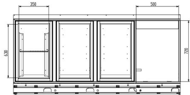
SEZIONE B-B
