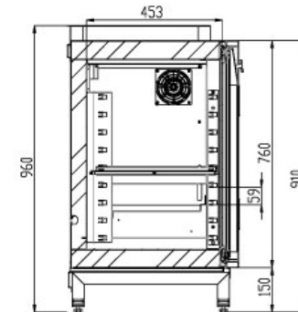
SEZIONE B-B
