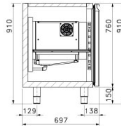
SEZIONE B-B
